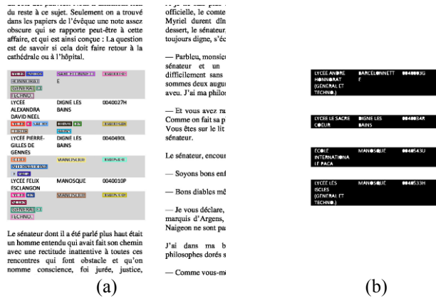
Figure 6: (a) les mots de la classe minoritaire sont entourés ; (b) les résultats de la croissance de région à partir des mots entourés dans l'image de gauche.
