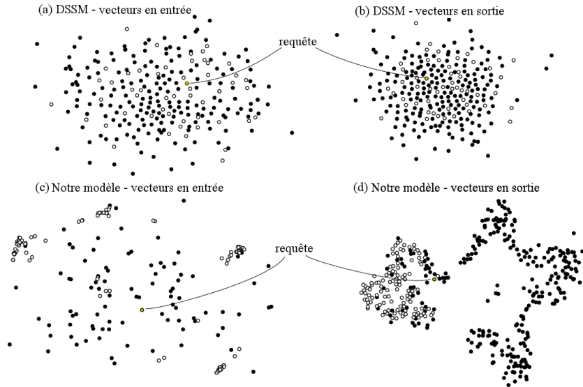
Figure 2. Analyse comparative de la projection t-SNE entre les vecteurs d'entrée (a)(c) et de sortie (b)(d) pour la requête 707 du jeu de données GOV2. \circ : documents pertinents - \bullet : documents non pertinents.
